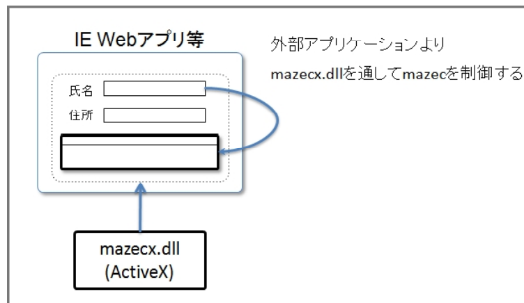
図 : mazec for Windows 概要図
