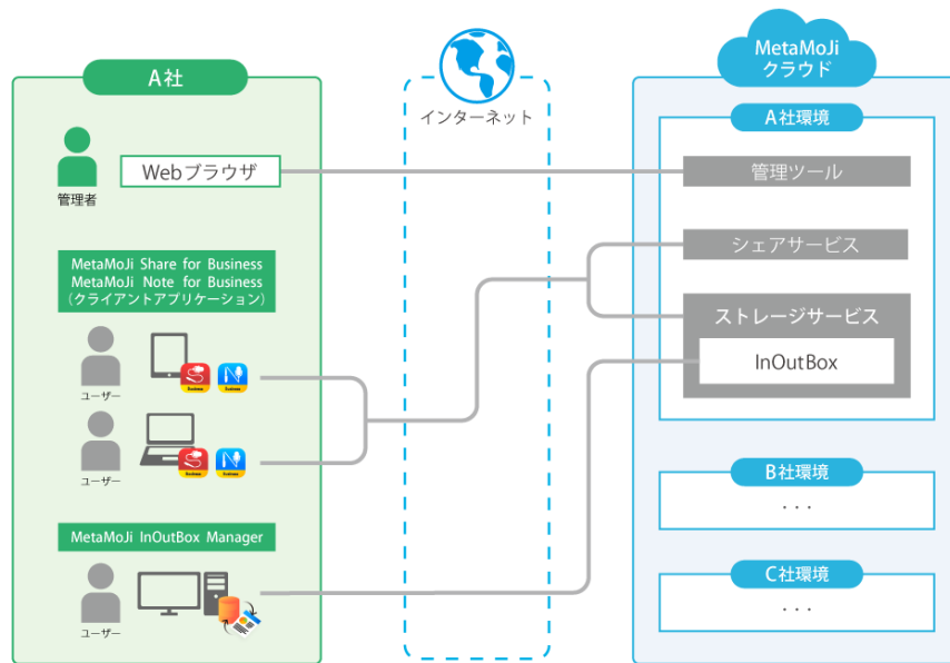
図：MetaMojI Share for Business・MetaMojI Note for Business システム構成
